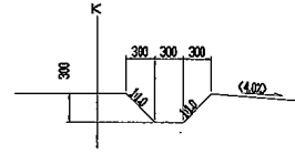
米堰水路断面図
